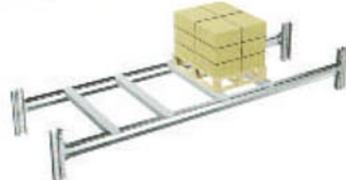
Tverrbjelker for lagring av pall ved langsideshåndtering.
