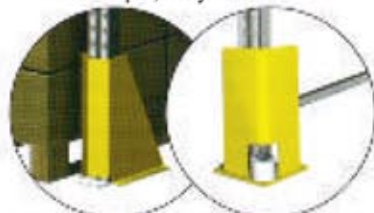
B. Påkjøringsbeskyttelse for stolpe, standard.
